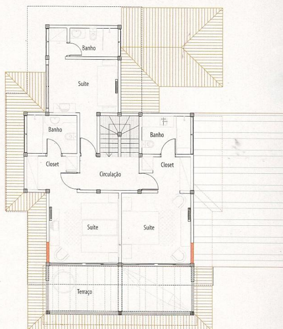
Planta Pavimento Superior
