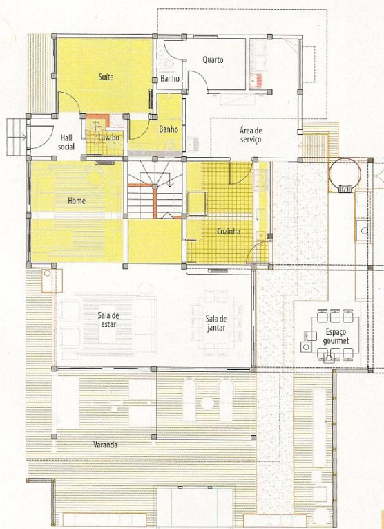
Planta Pavimento Térreo
